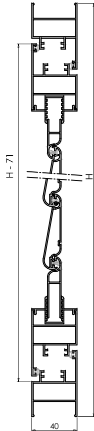
SECCION B - B'
