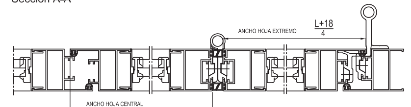
Sección lateral de ventana de 4 hojas
