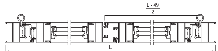
Sección A-A'
