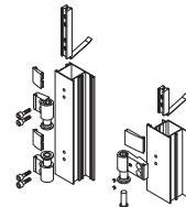
4029 Bisagra 3 alas puerta Apertura Externa
