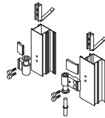
4027 Bisagra puerta Apertura Externa
