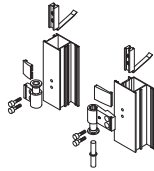
4026 Bisagra puerta Apertura Interna
