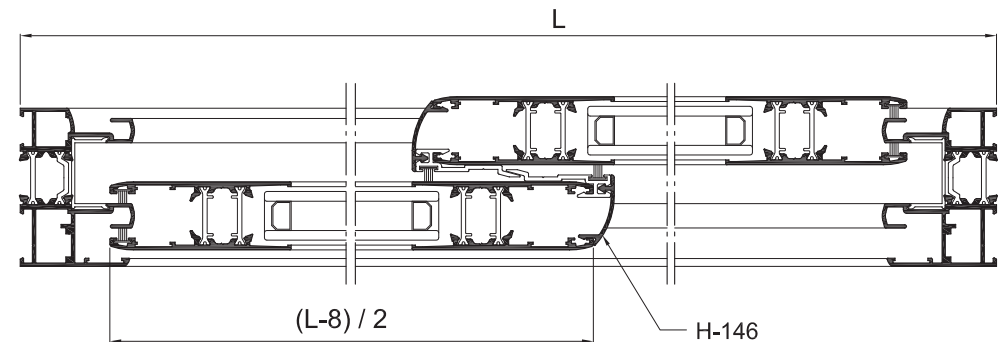
Sección A-A'
