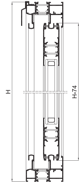
Sección B-B'
