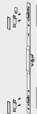
4189 Cierre multipunto H > 1869
