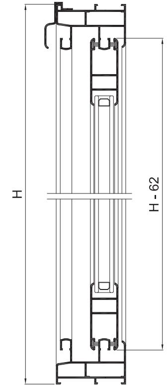
Sección B-B'
