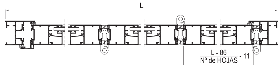
Sección A-A'
