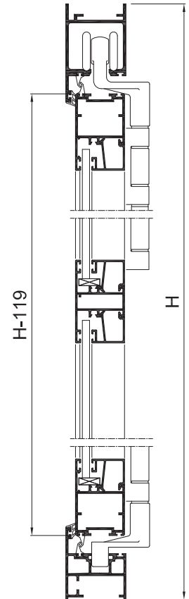
Sección B-B'
