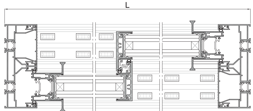
Sección A-A'
