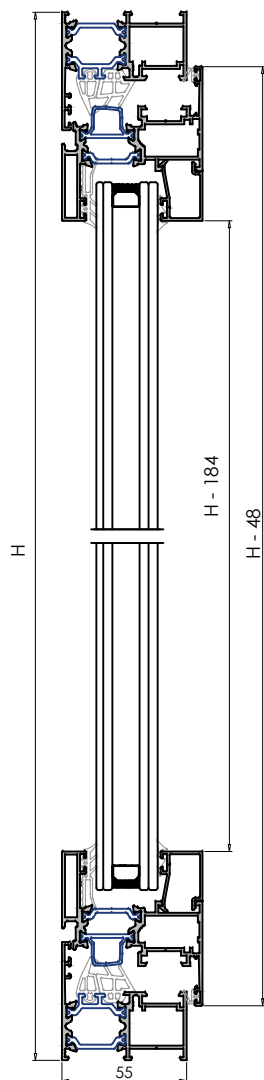
SECCION B - B'
