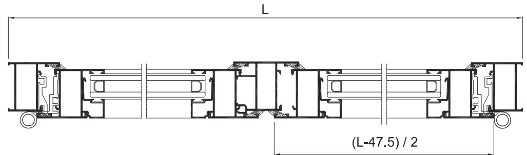
Sección A-A'
